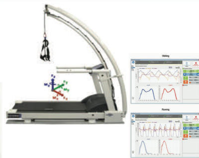
三維步態跑步機
