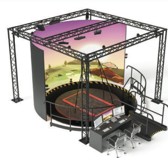
虛擬場景六軸平台
